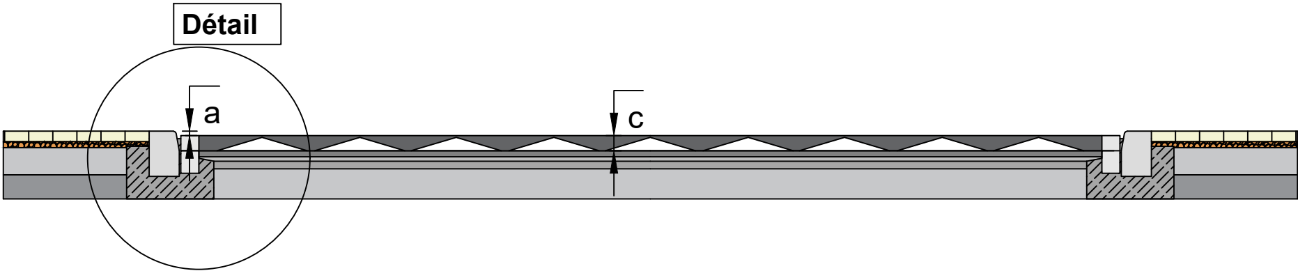
Coupe A-A
